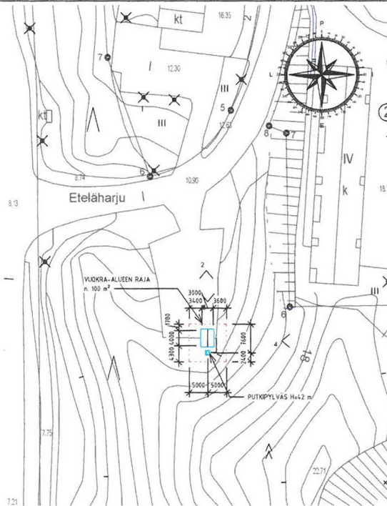
Asemapiirros 1_500 1: 500
