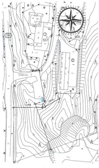
Asemapiirros 1_1000 1: 1000
