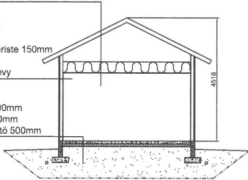
Leikkaus
