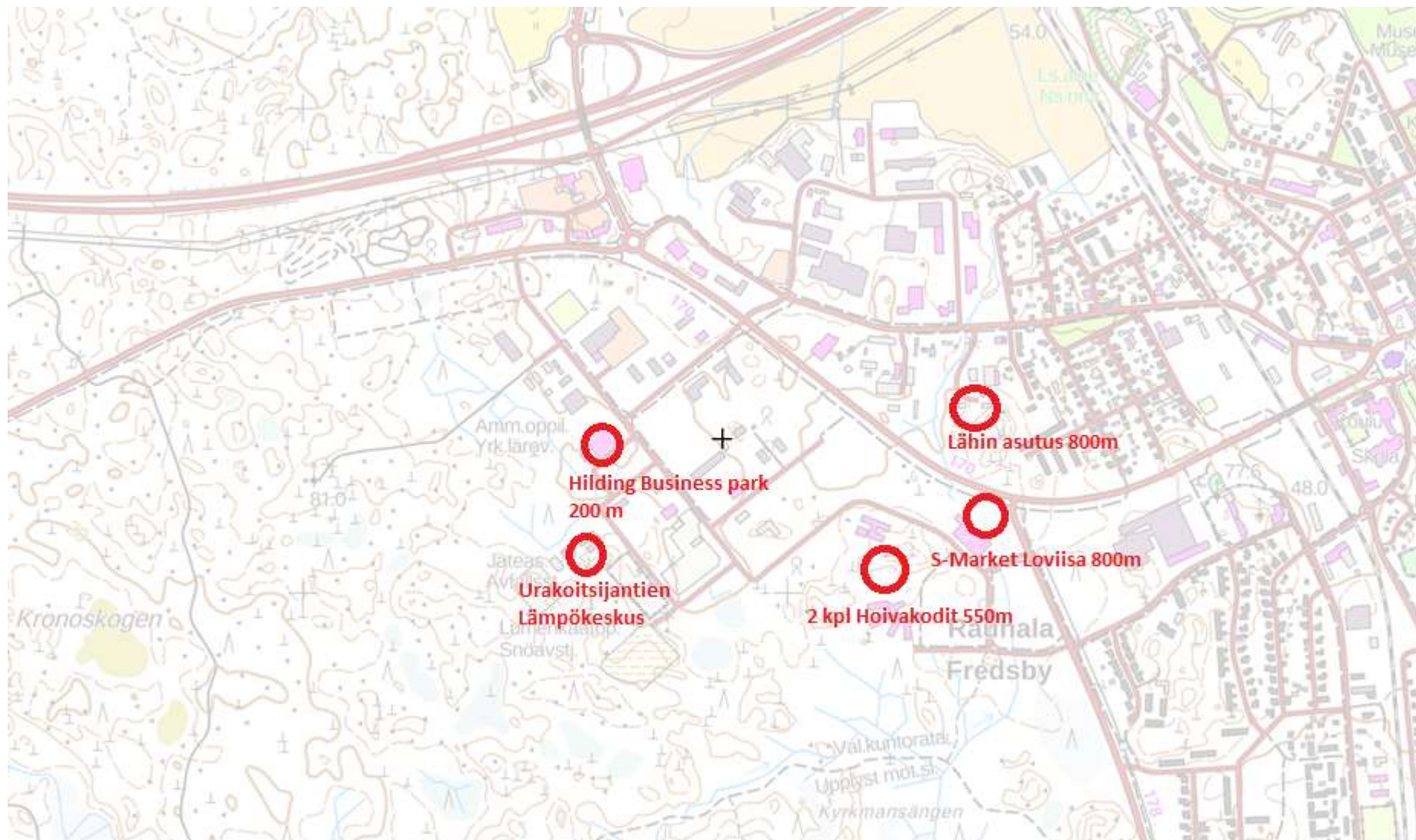
Liite 1. Urakoitsijantien Lämpökeskus ja lähimmät häiriintyvät kohteet
