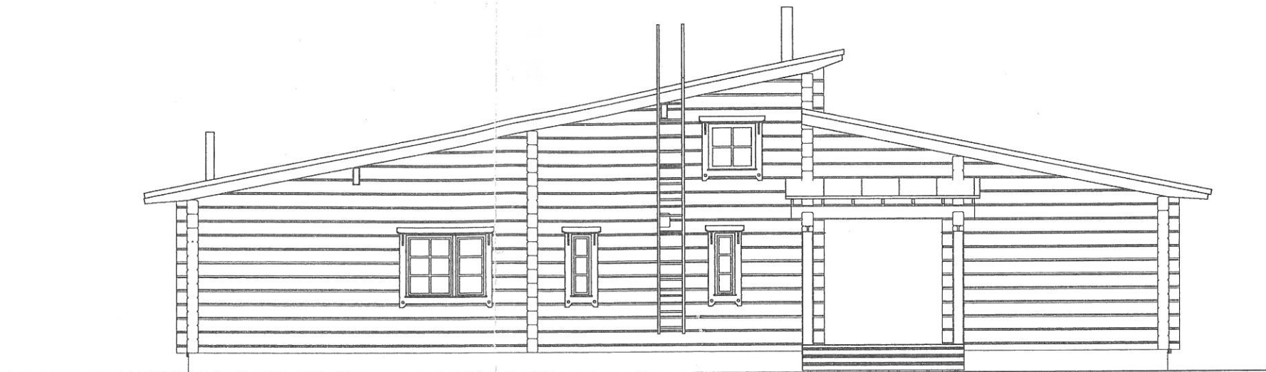
JULKISIVU 3
