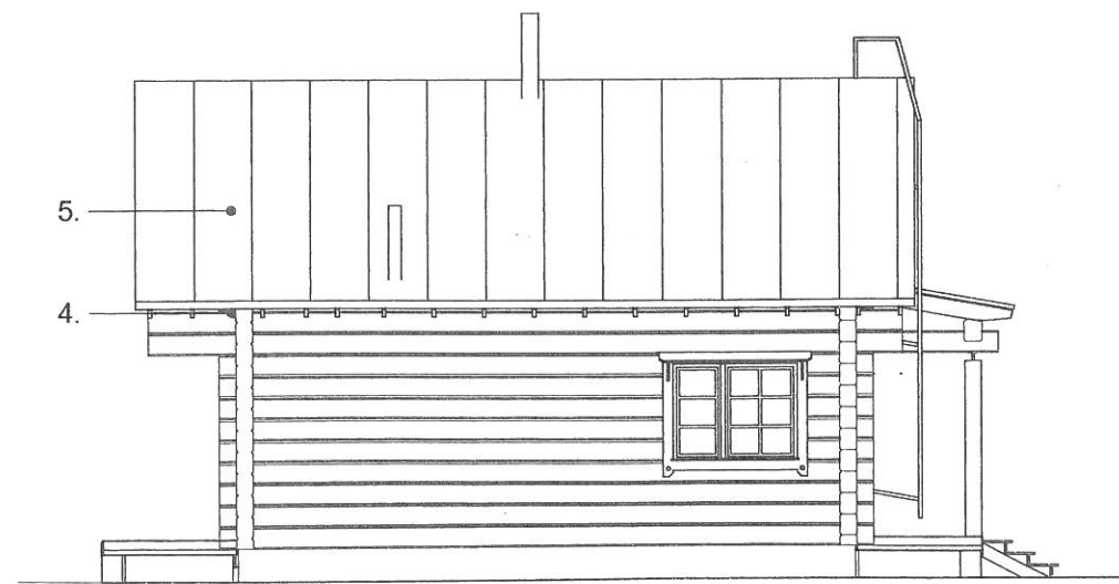
JULKISIVU 2
