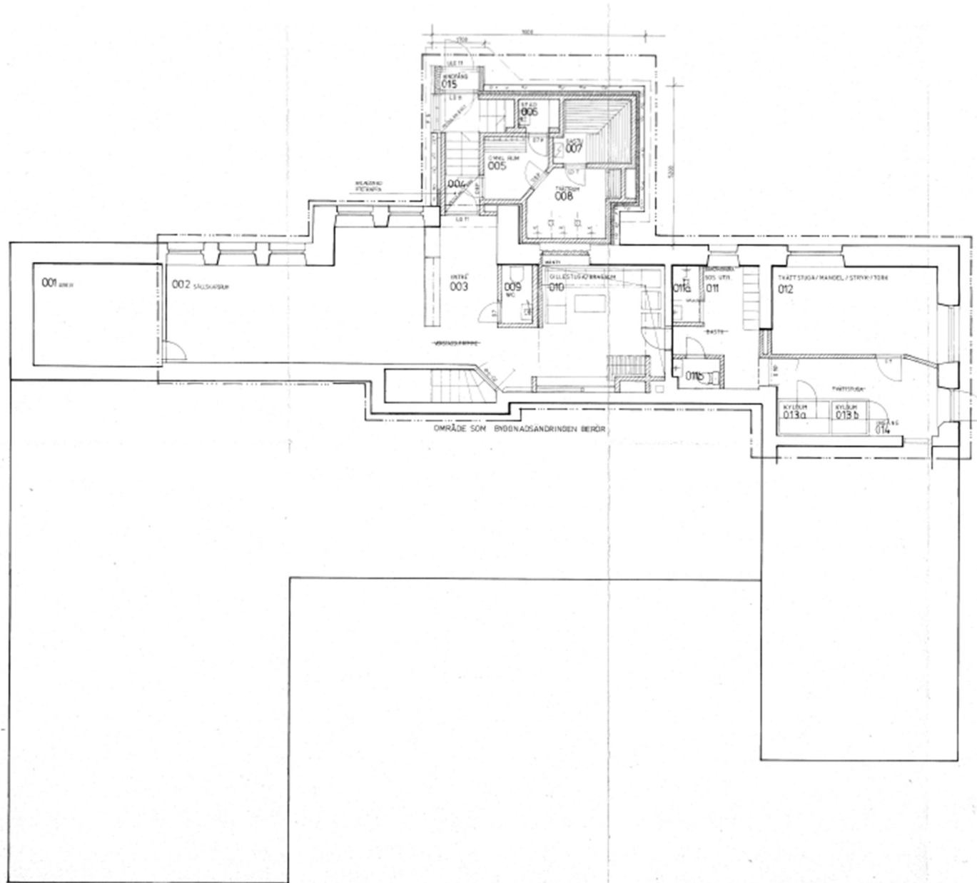
Kuva 7. Päärakennuksen kellarikerros.
