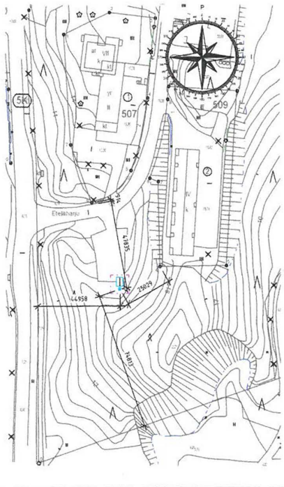
Asemapiirros 1_1000 1: 1000
