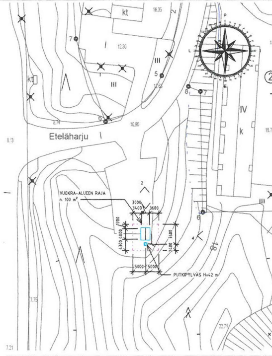
Asemapiirros 1_500 1: 500
