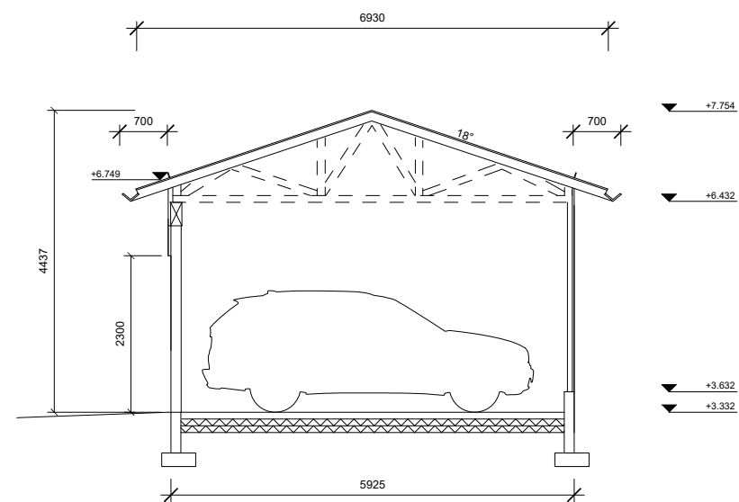
Leikkaus B-B
