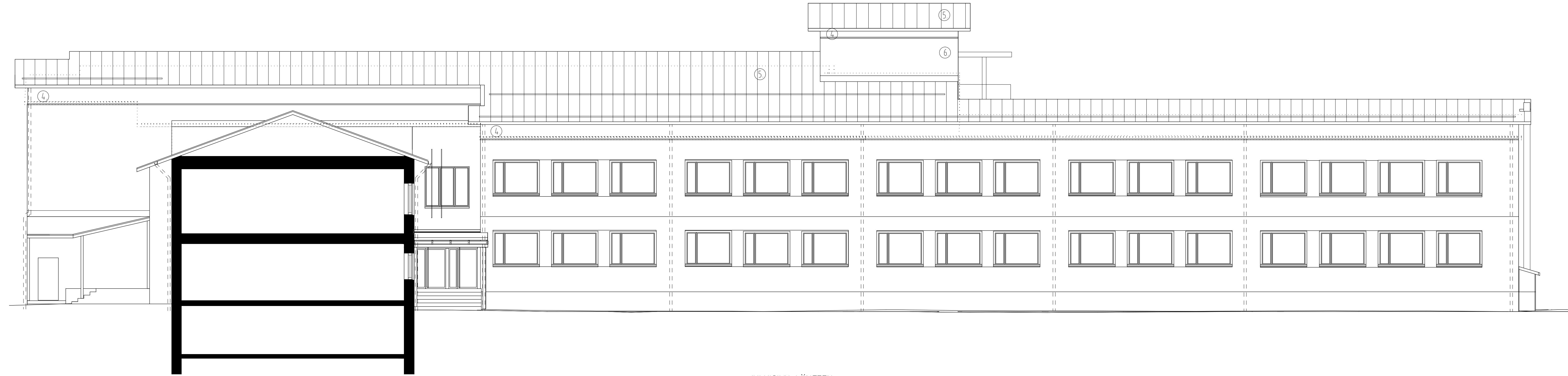
JULKISIVU LÄNTEEN
