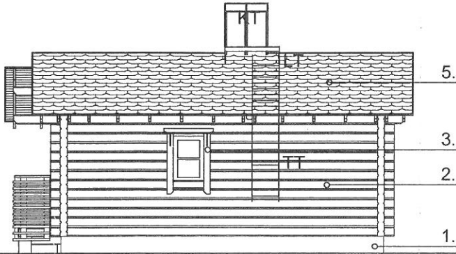
JULKISIVU 3
