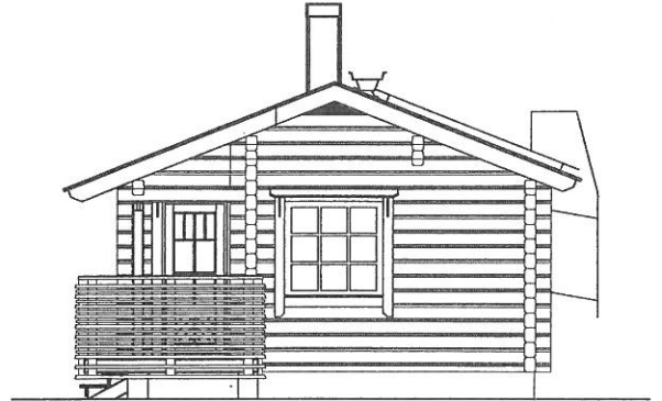
JULKISIVU 4
