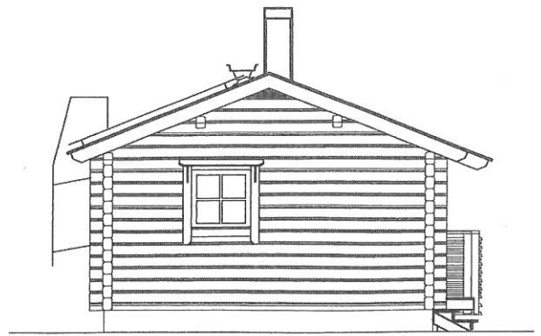
JULKISIVU 2
