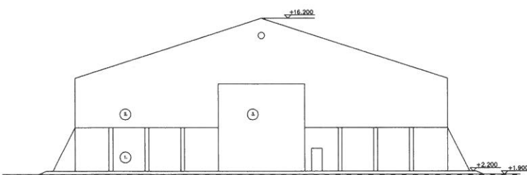
JULKISIVU LOUNAASEEN
