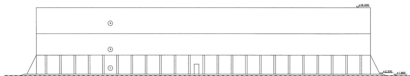
JULKISIVU KAAKKOON
